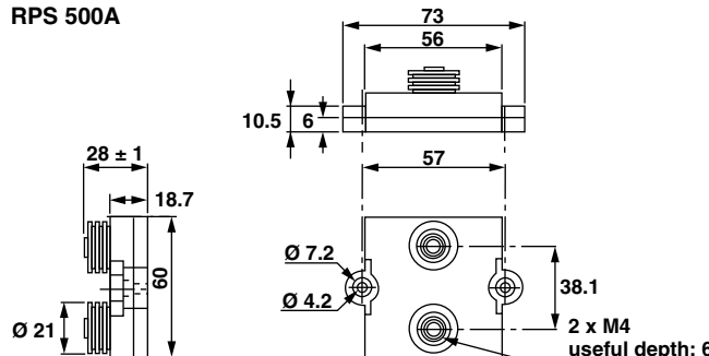
RPS 500A
