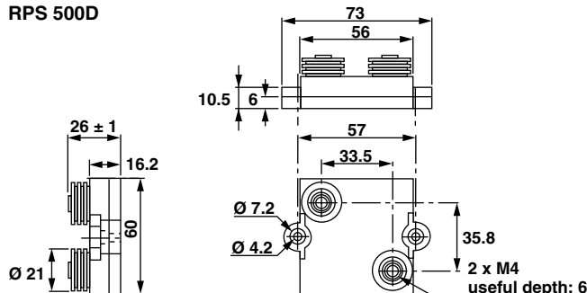
RPS 500D
